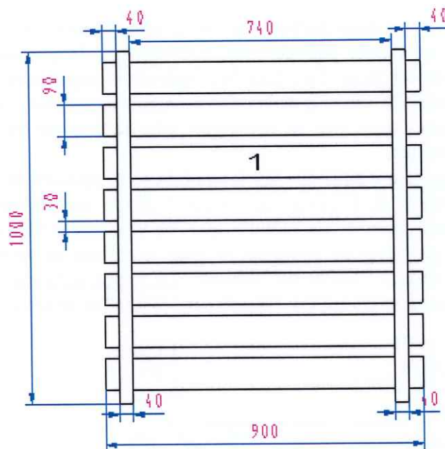
Plan du panneau arrière
